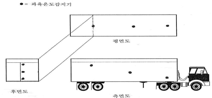
[그림 1] 컨테이너 저온처리 시 과육 온도 감지용 센서 설치 위치도
